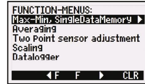
Function menus
